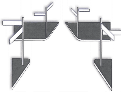
FIG.291 art.133 SEGNALE NOME STRADA APPLICATO IN ANGOLO
