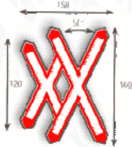
FIG.10/d art.87 CROCE DI S.ANDREA INSTALLATA VERTICALMENTE
