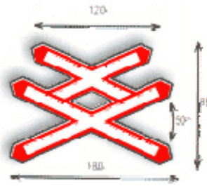
FIG.10/b art.87 DOPPIA CROCE DI S.ANDREA
